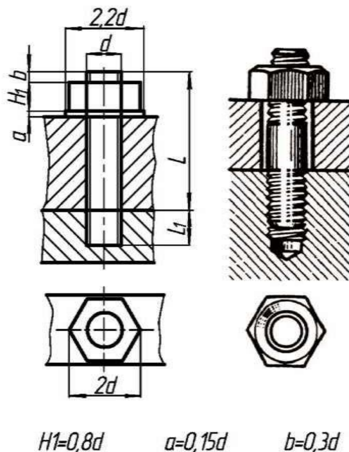
Рис. 3. Упрощенное изображение шпилечного соединения
