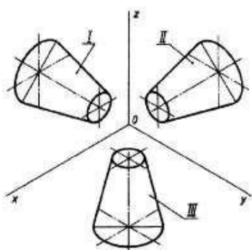
Рис. 96. Усеченные конусы
