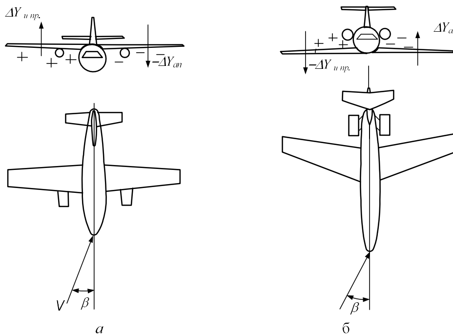
Рисунок 6.11 – Скольжение и крен высокоплана и низкоплана
