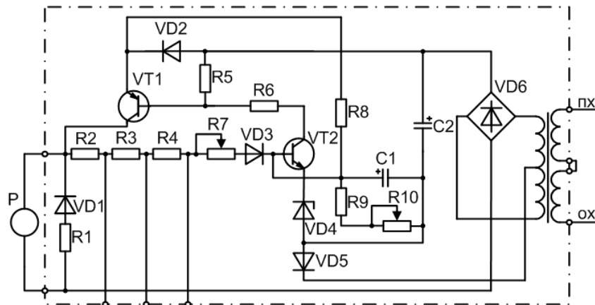
Рисунок 1. Схема РНП
